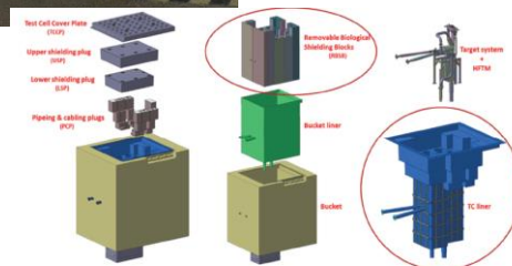
Ilustración 2 Concepto mantenedor de la Test Cell de IFMIF-DONES
